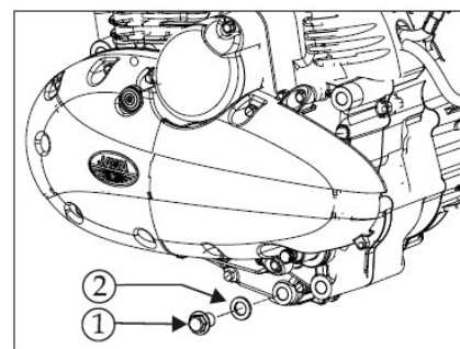
(1) vypouštěcí šroub (2) těsnící podložka
