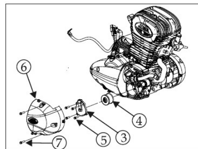
(3) víčko olejového filtru (4) olejový filtr (5) šroub víka (6) kryt (7) šroub
